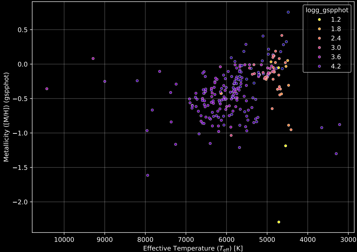
GALAH DR4 Field: [7226] Stellar Population Parameters (n= 234)
